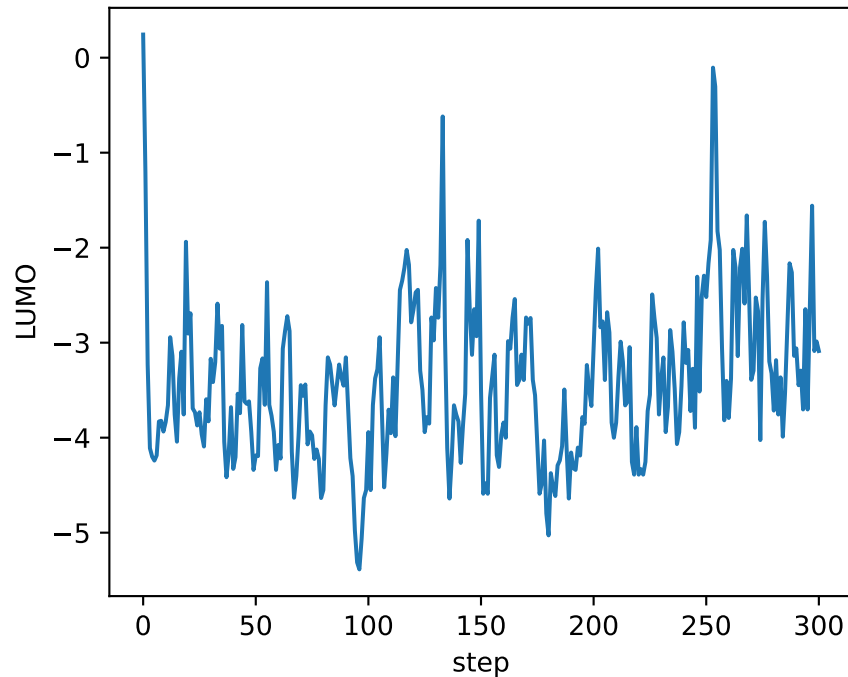
LUMO - evolution
